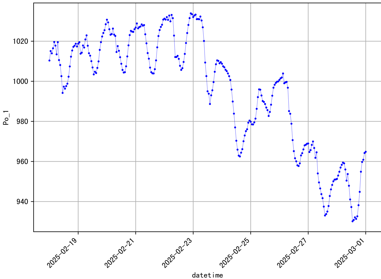
'H' data (11 days, 59 min/dp) 105166@105166EA_Po_1
