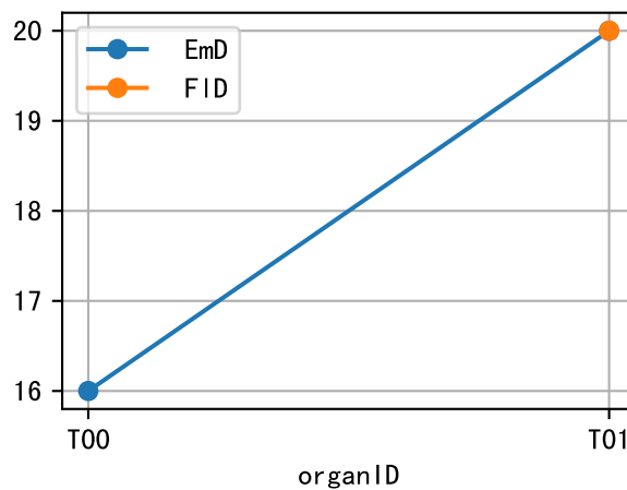
EQ2AW-49-6 Phe
