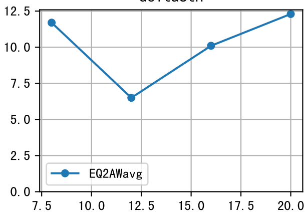
deltaStH
