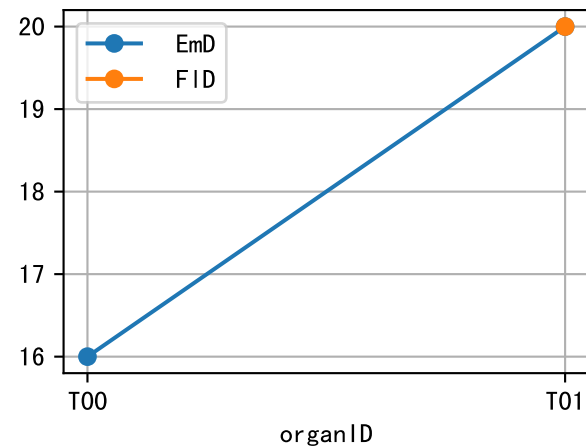
EQ2AW-38-31 Phe
