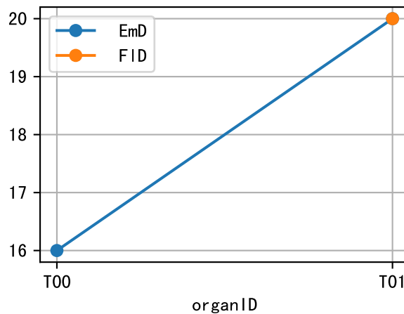
EQ2AW-32-58 Phe
