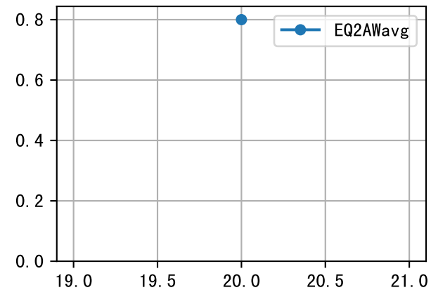
TsNR
