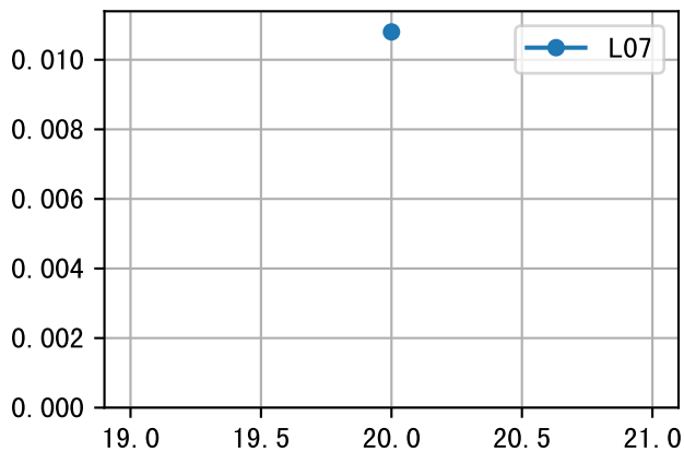
LfA (EQ2AW-32-58)
