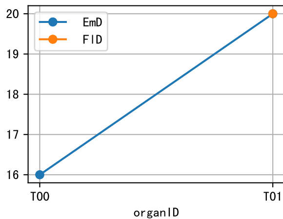
EQ2AW-41-47 Phe
