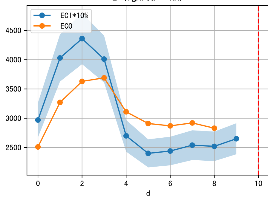
2 (fgArea = NA)
