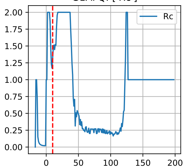
G1AFQ: ['Rc']
