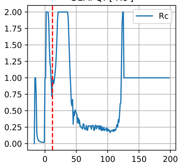
G1AFQ: ['Rc']
