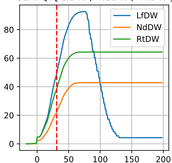
G1AFQ: ['LfDW', 'NdDW', 'RtDW']
