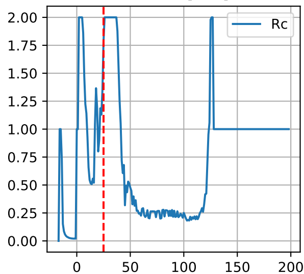
G1AXG: ['Rc']
