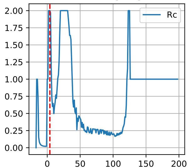
G1AXG: ['Rc']
