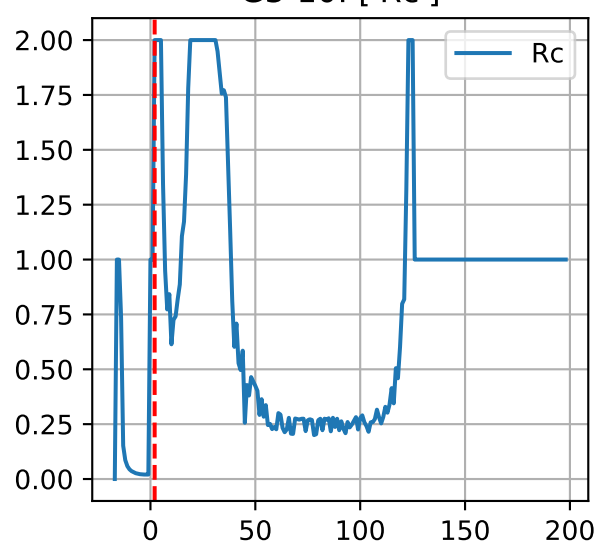
G3-10: ['Rc']
