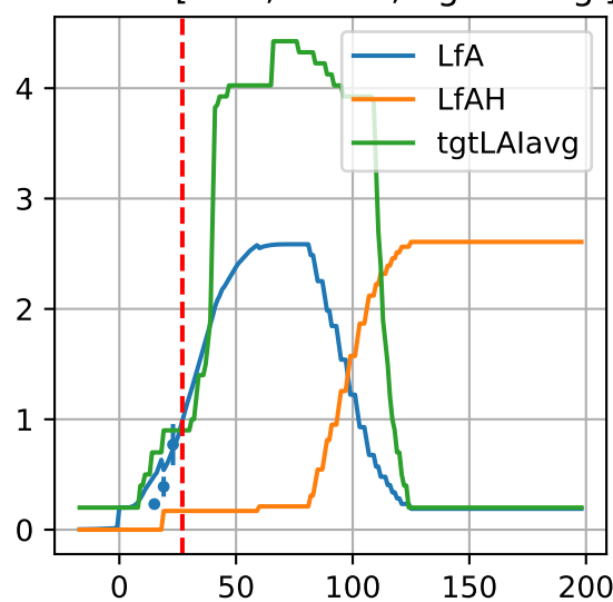
G3-11: ['LfA', 'LfAH', 'tgtLAlavg']
