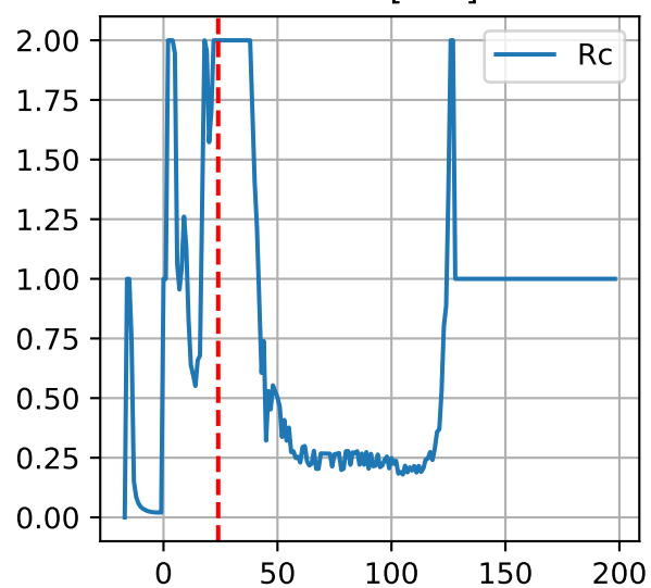
G3-12: ['Rc']
