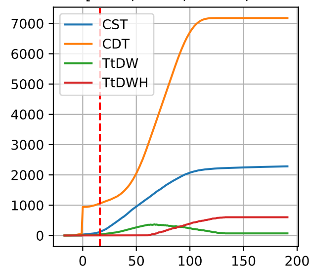
G3-15: ['CST', 'CDT', 'TtDW', 'TtDWH']
