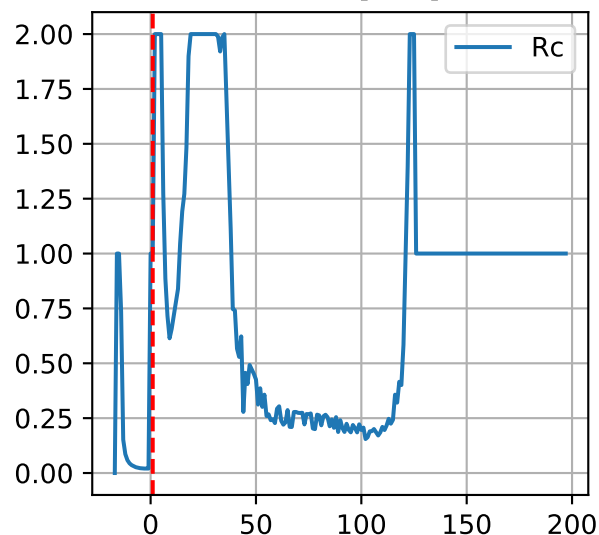
G3-16: ['Rc']
