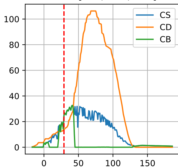
G3-1: ['CS', 'CD', 'CB']
