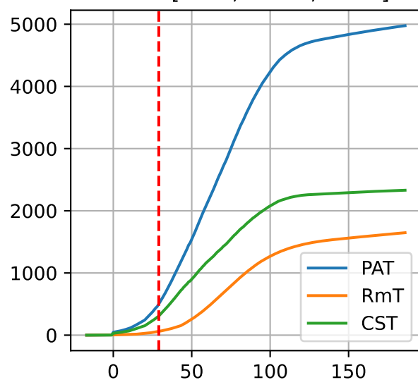
G3-1: ['PAT', 'RmT', 'CST']
