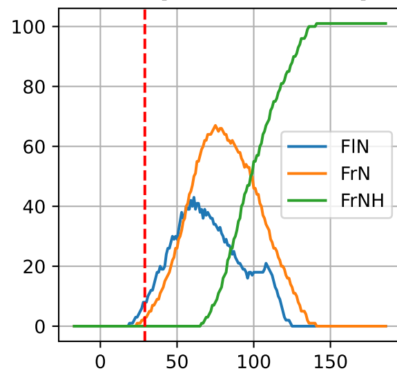
G3-1: ['FIN', 'FrN', 'FrNH']
