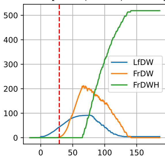
G3-1: ['LfDW', 'FrDW', 'FrDWH']
