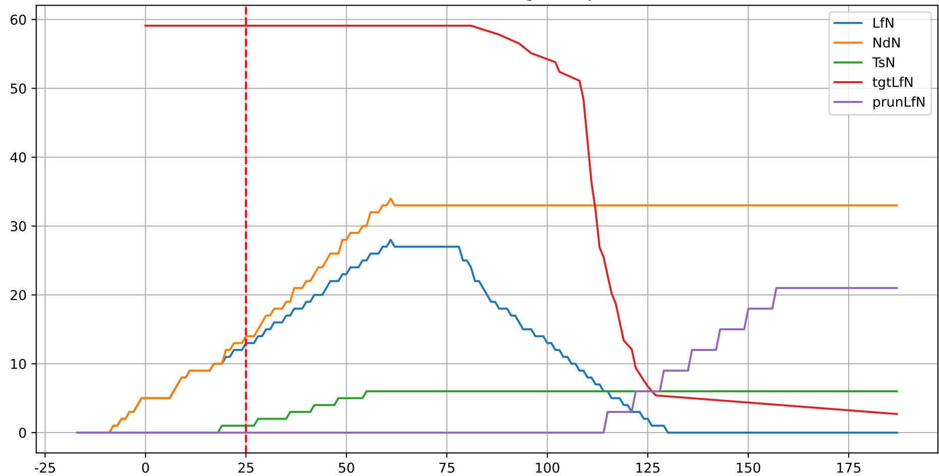
G3-5: ['LfN', 'NdN', 'TsN', 'tgtLfN', 'prunLfN']
