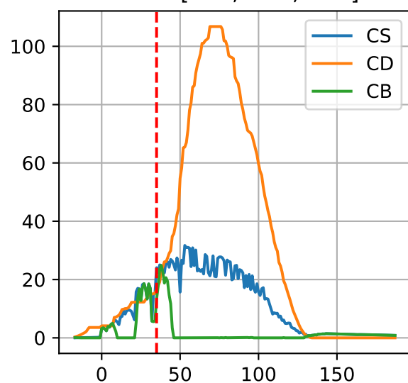
G3-5: ['CS', 'CD', 'CB']
