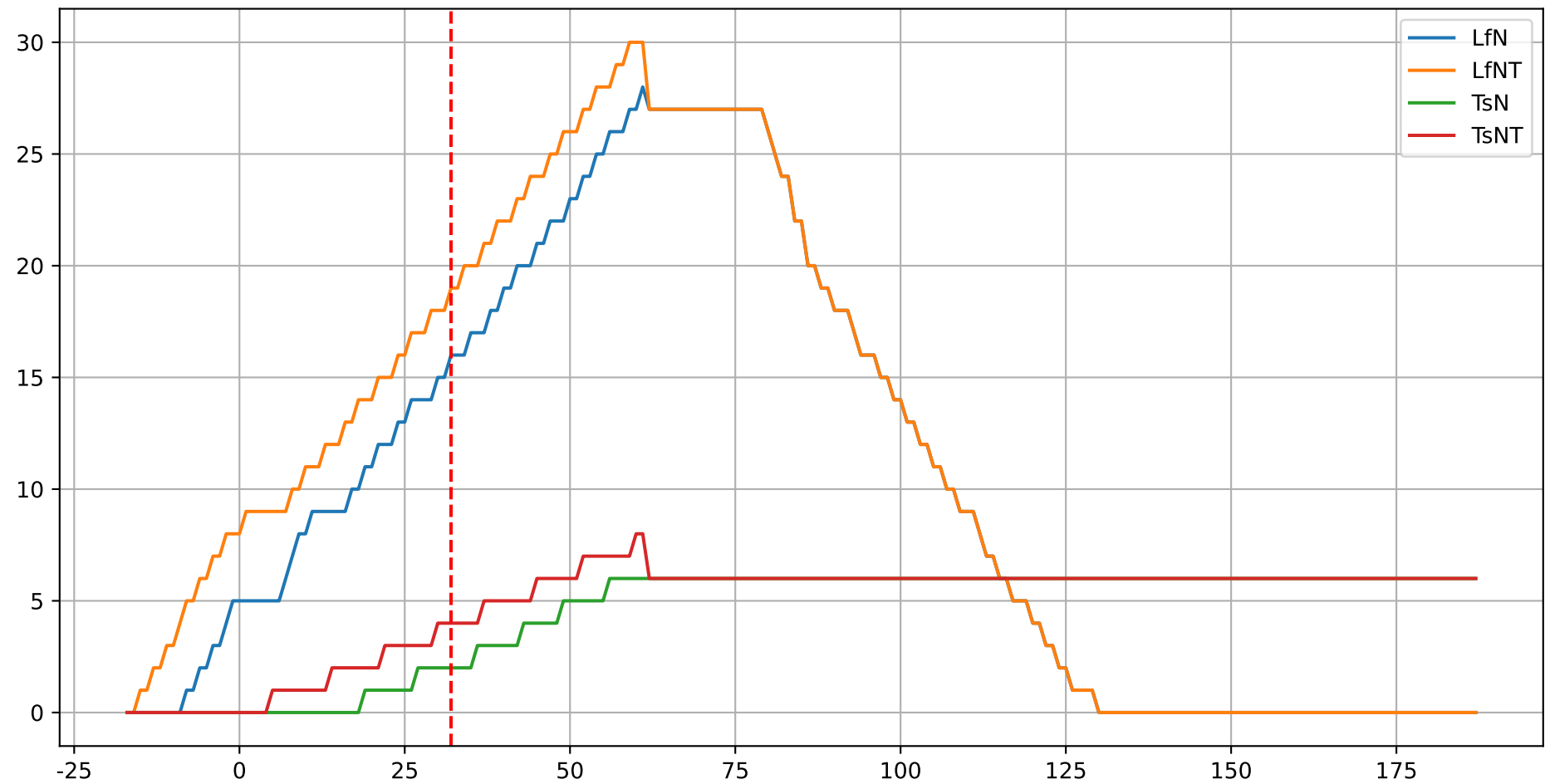
G3-6: ['LfN', 'LfNT', 'TsN', 'TsNT']
