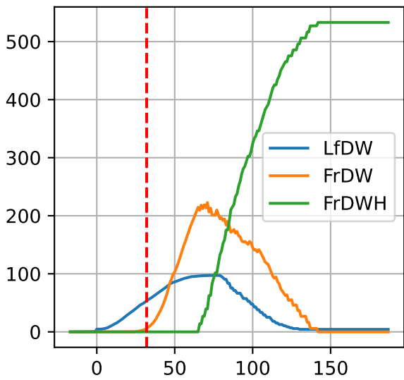
G3-6: ['LfDW', 'FrDW', 'FrDWH']
