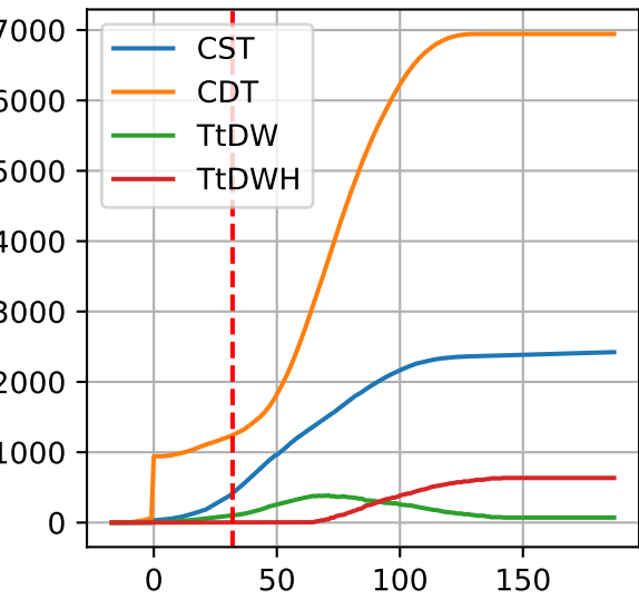
G3-6: ['CST', 'CDT', 'TtDW', 'TtDWH']
