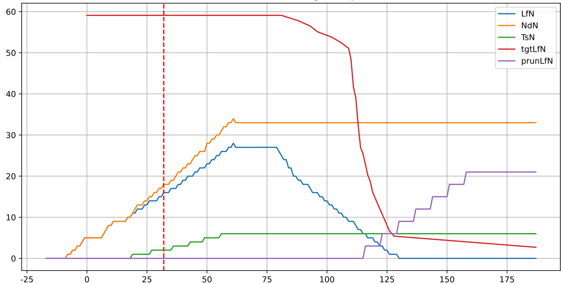
G3-6: ['LfN', 'NdN', 'TsN', 'tgtLfN', 'prunLfN']
