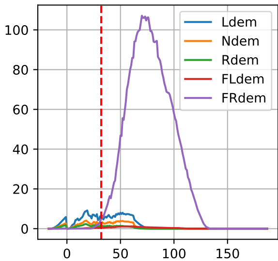
G3-6: ['Ldem', 'Ndem', 'Rdem', 'FLdem', 'FRdem']
