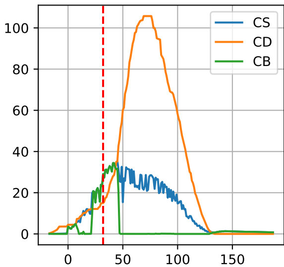
G3-6: ['CS', 'CD', 'CB']
