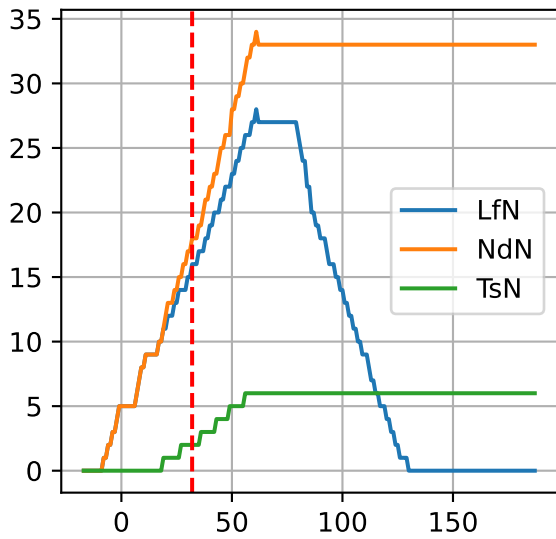
G3-6: ['LfN', 'NdN', 'TsN']
