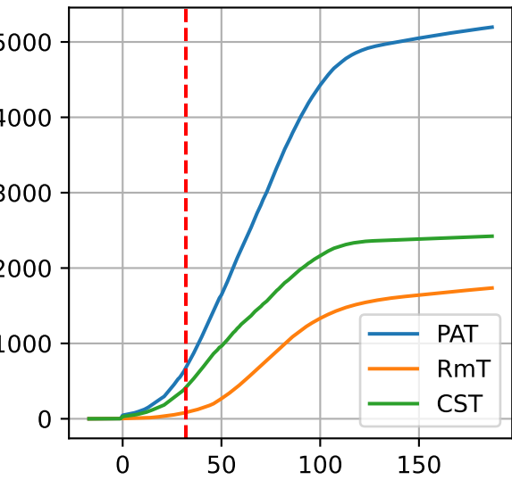
G3-6: ['PAT', 'RmT', 'CST']
