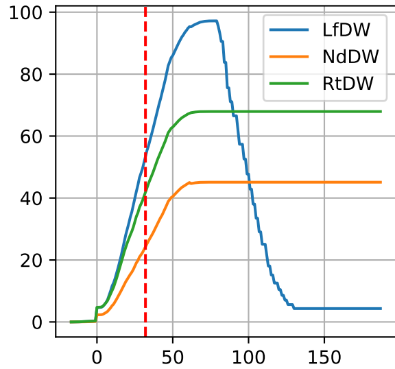
G3-6: ['LfDW', 'NdDW', 'RtDW']
