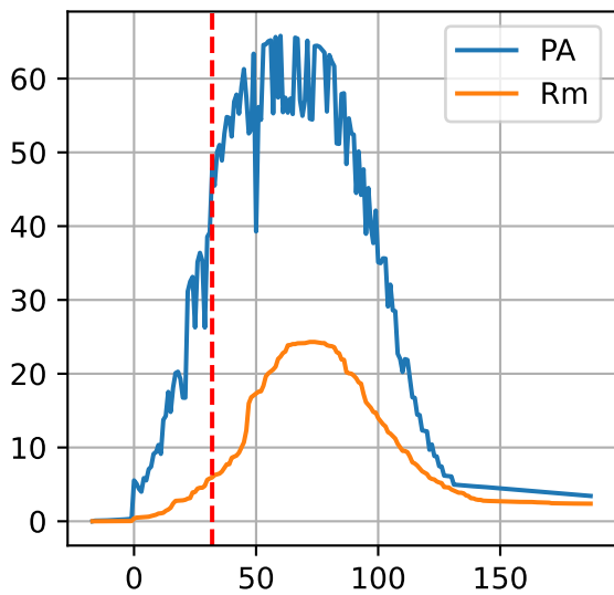
G3-6: ['PA', 'Rm']
