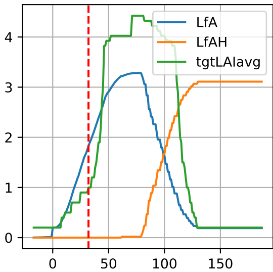
G3-6: ['LfA', 'LfAH', 'tgtLAlavg']
