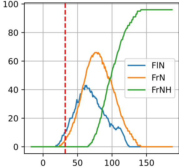
G3-6: ['FIN', 'FrN', 'FrNH']
