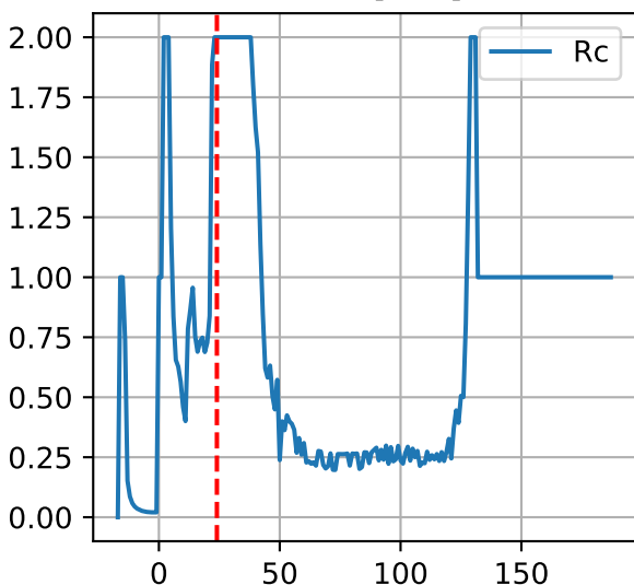
G3-7: ['Rc']
