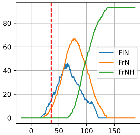
G3-8: ['FIN', 'FrN', 'FrNH']
