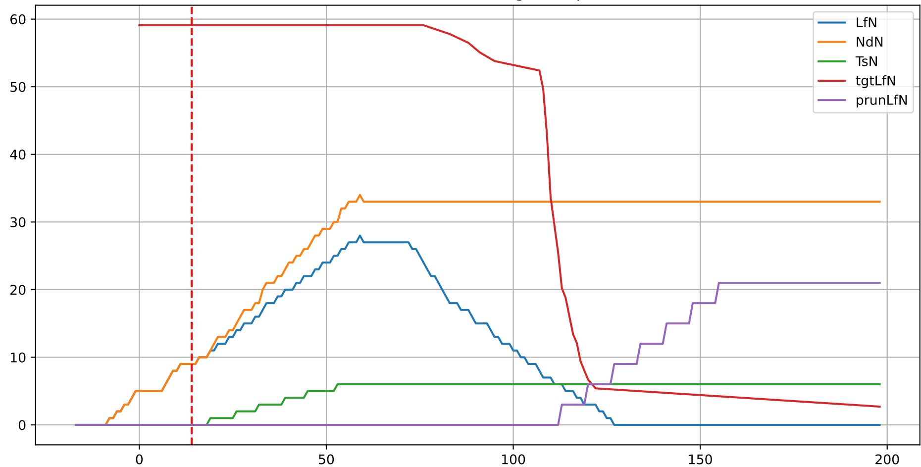
G3-9: ['LfN', 'NdN', 'TsN', 'tgtLfN', 'prunLfN']
