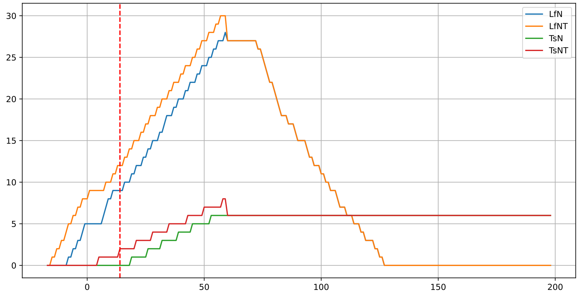
G3-9: ['LfN', 'LfNT', 'TsN', 'TsNT']
