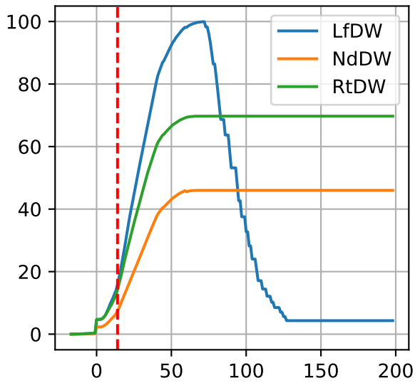
G3-9: ['LfDW', 'NdDW', 'RtDW']
