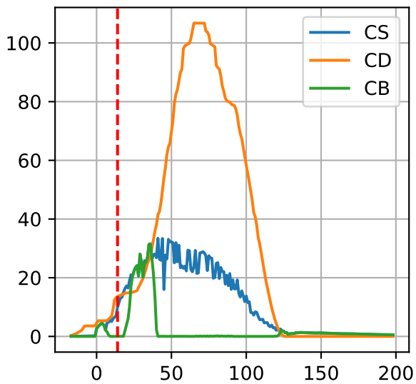
G3-9: ['CS', 'CD', 'CB']
