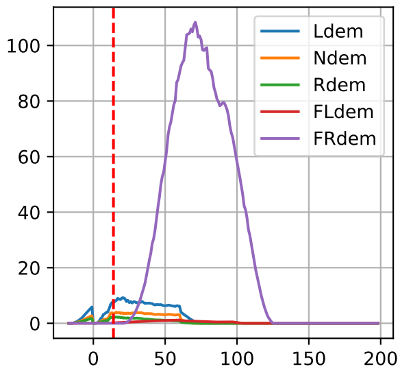
G3-9: ['Ldem', 'Ndem', 'Rdem', 'FLdem', 'FRdem']
