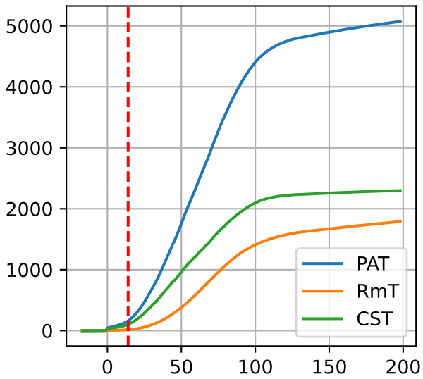
G3-9: ['PAT', 'RmT', 'CST']
