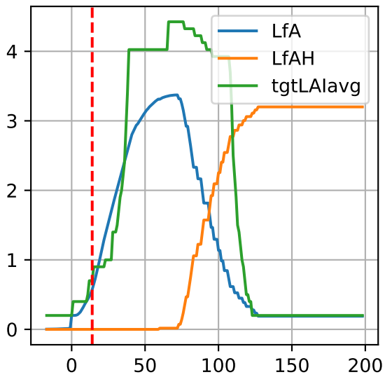
G3-9: ['LfA', 'LfAH', 'tgtLAlavg']
