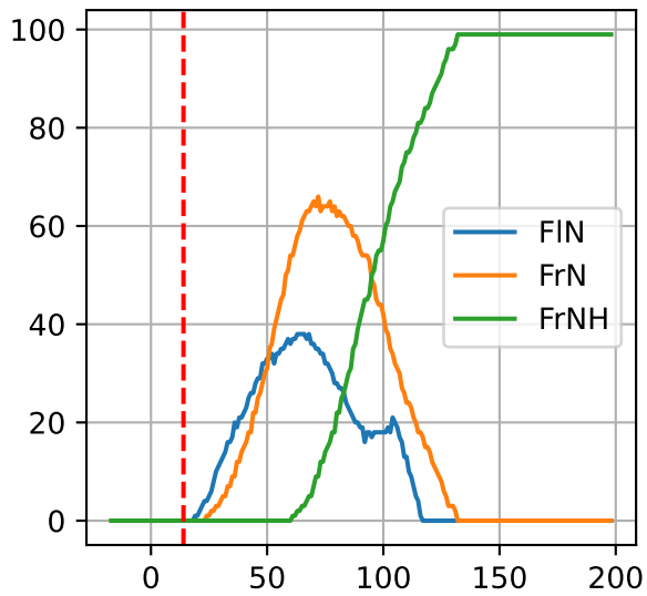
G3-9: ['FIN', 'FrN', 'FrNH']
