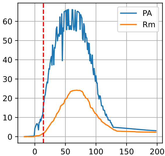
G3-9: ['PA', 'Rm']
