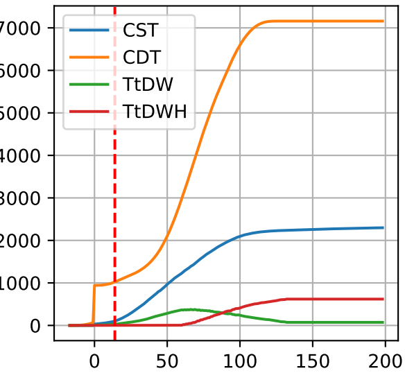
G3-9: ['CST', 'CDT', 'TtDW', 'TtDWH']
