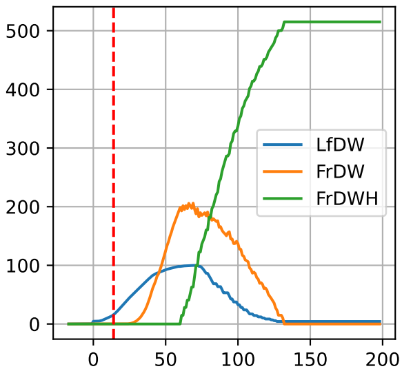
G3-9: ['LfDW', 'FrDW', 'FrDWH']
