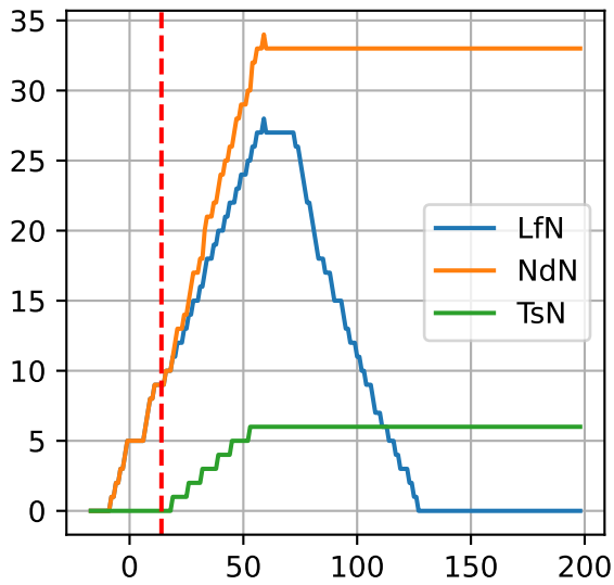
G3-9: ['LfN', 'NdN', 'TsN']
