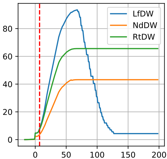
G3-9: ['LfDW', 'NdDW', 'RtDW']
