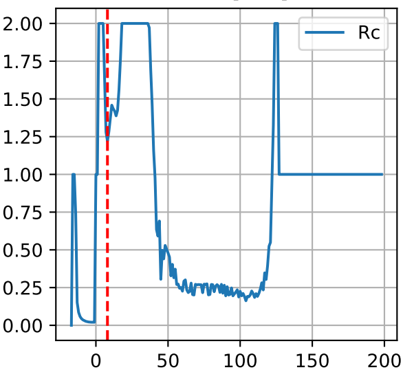
G3-9: ['Rc']
