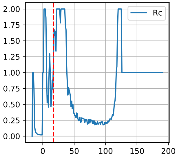
G4: ['Rc']
