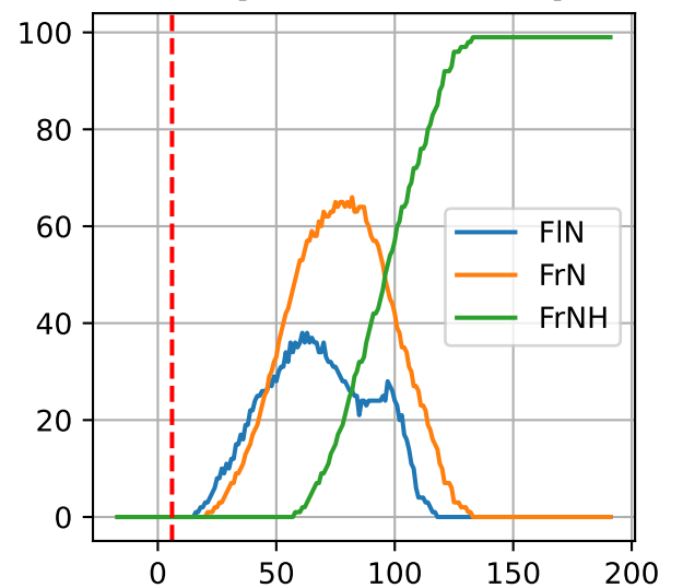
G4: ['FIN', 'FrN', 'FrNH']
