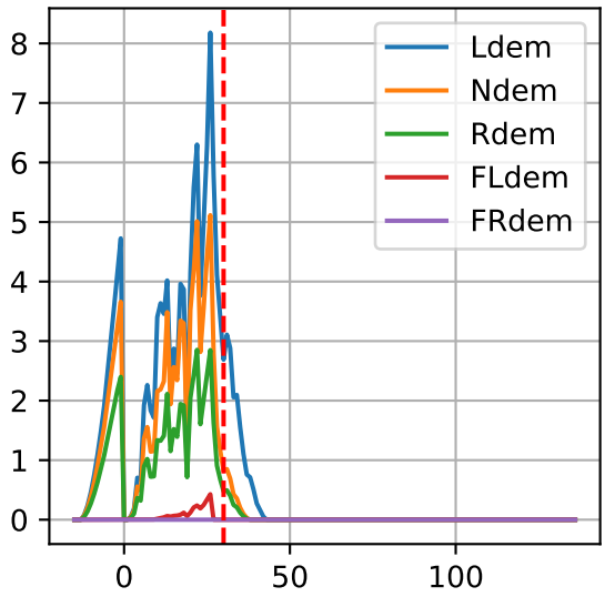
M2: ['Ldem', 'Ndem', 'Rdem', 'FLdem', 'FRdem']
