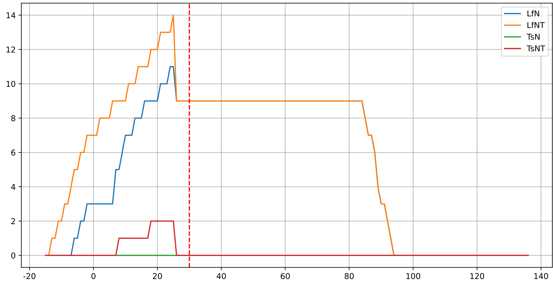
M2: ['LfN', 'LfNT', 'TsN', 'TsNT']
