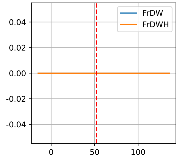
M2: ['FrDW', 'FrDWH', 'adjFrDW', 'adjFrDWH']
