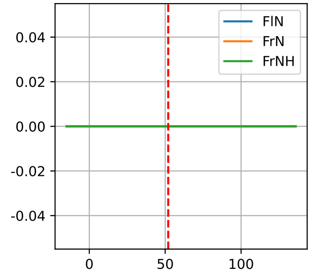
M2: ['FIN', 'FrN', 'FrNH']
