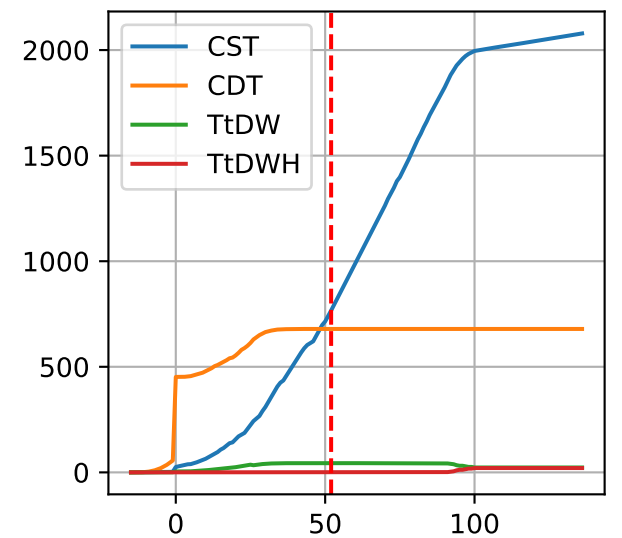
M2: ['CST', 'CDT', 'TtDW', 'TtDWH']
