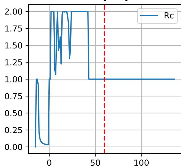
M2: ['Rc']
