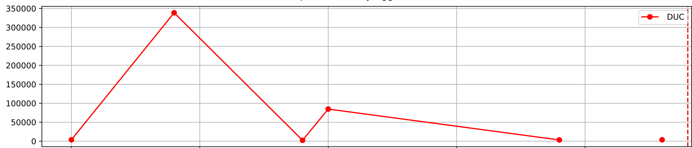
plot dfFv (daily Agg)
