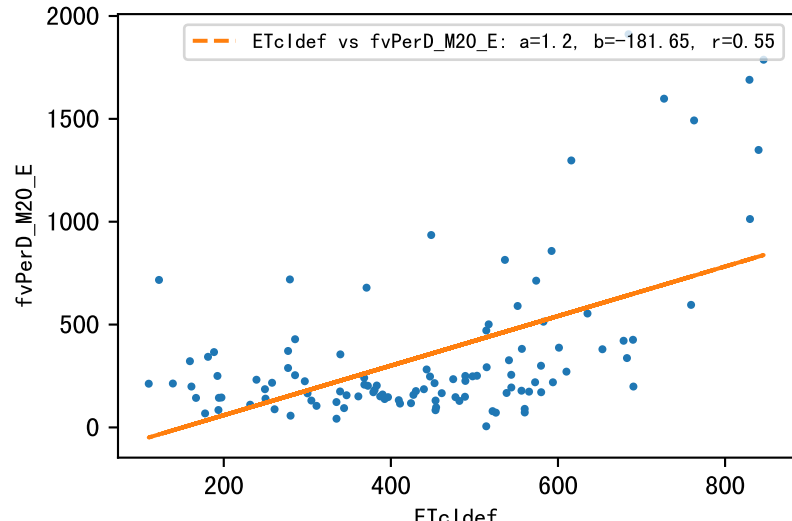
M20_E ETcldef vs estFv
