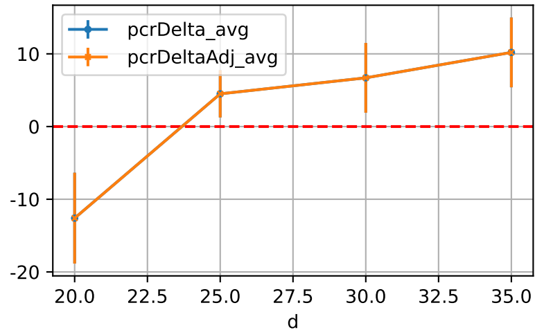
DeltaTypeAbbr=GrpByDay
