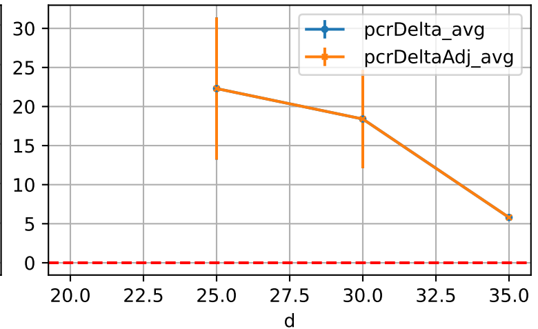
DeltaTypeAbbr=WeiAvgByD
