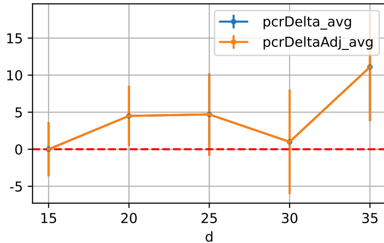
DeltaTypeAbbr=GrpByAge
