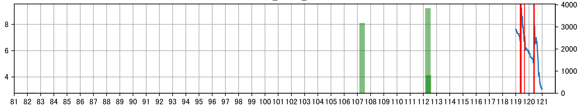
P10AW_W1: M_E40
