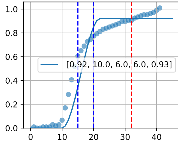
M_W d43 ([40.0, 17.9, -7.0] fdu=20.0)
