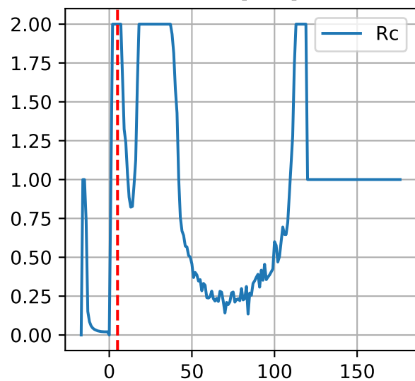
P11: ['Rc']
