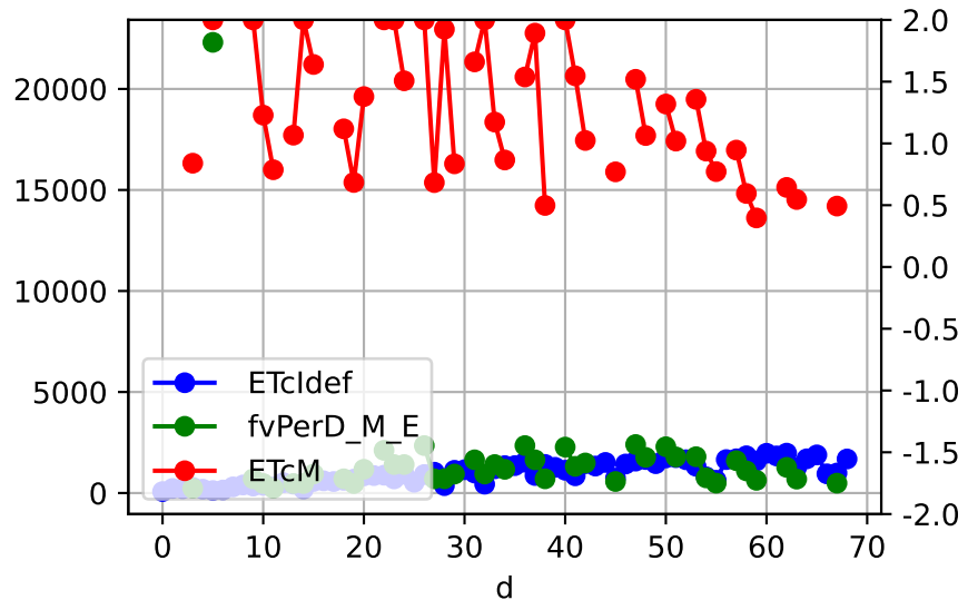
M_E ETcldef vs estFv
