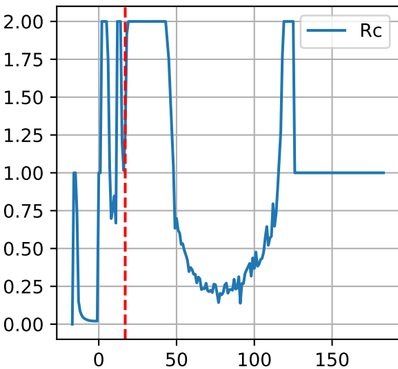
P12: ['Rc']
