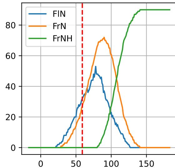
P12: ['FIN', 'FrN', 'FrNH']
