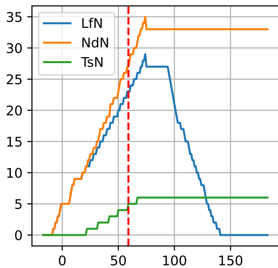
P12: ['LfN', 'NdN', 'TsN']
