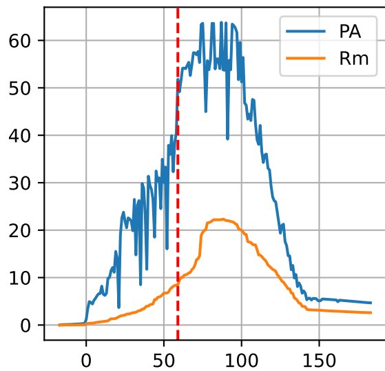
P12: ['PA', 'Rm']
