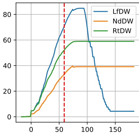
P12: ['LfDW', 'NdDW', 'RtDW']
