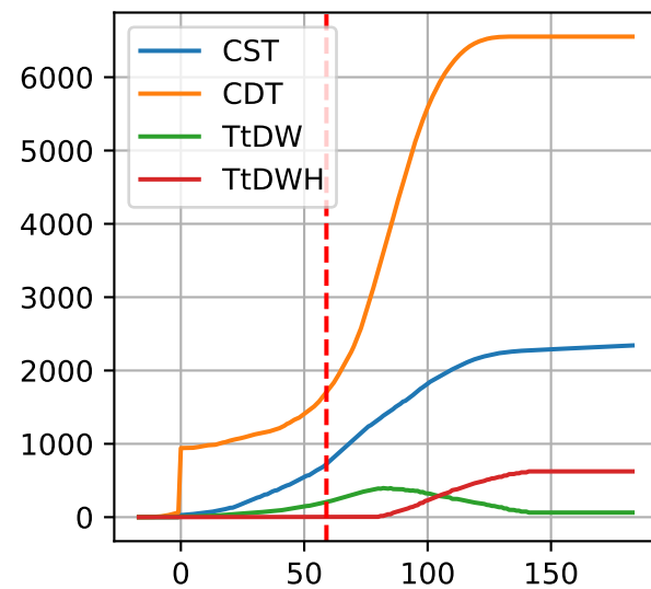
P12: ['CST', 'CDT', 'TtDW', 'TtDWH']
