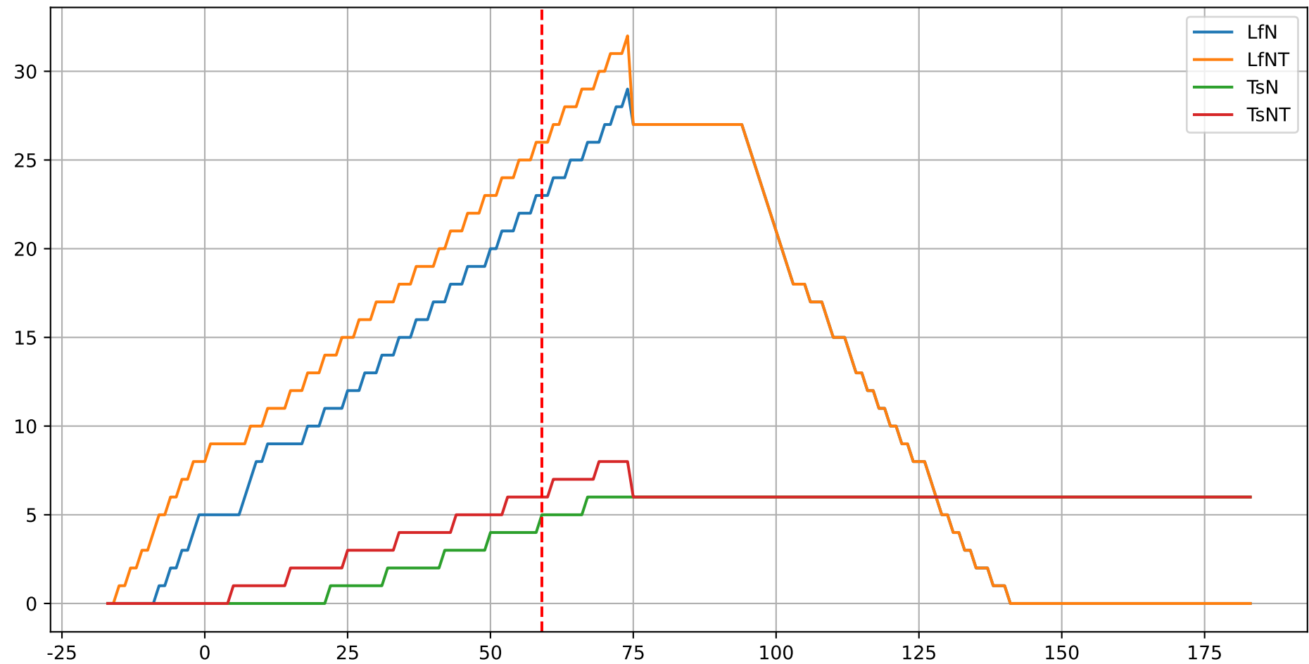
P12: ['LfN', 'LfNT', 'TsN', 'TsNT']
