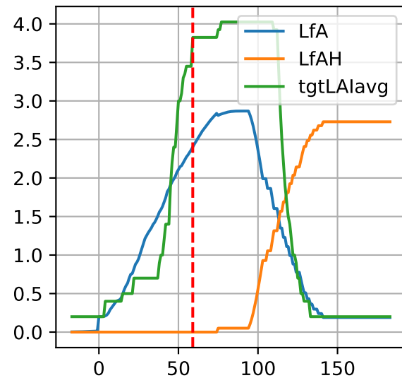
P12: ['LfA', 'LfAH', 'tgtLAlavg']
