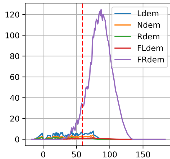
P12: ['Ldem', 'Ndem', 'Rdem', 'FLdem', 'FRdem']
