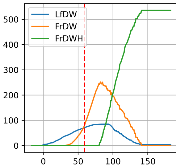
P12: ['LfDW', 'FrDW', 'FrDWH']
