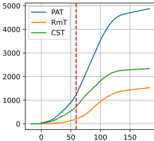
P12: ['PAT', 'RmT', 'CST']
