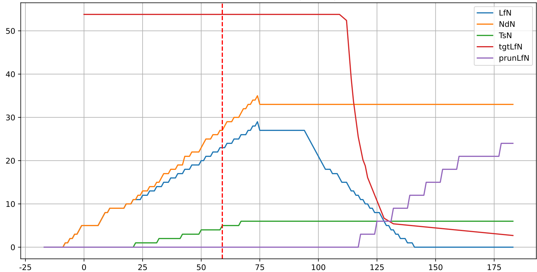
P12: ['LfN', 'NdN', 'TsN', 'tgtLfN', 'prunLfN']
