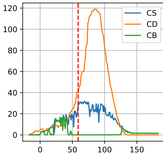
P12: ['CS', 'CD', 'CB']
