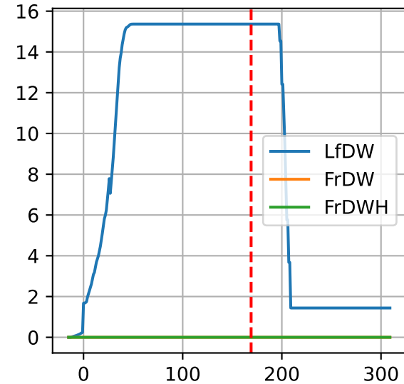
P1: ['LfDW', 'FrDW', 'FrDWH']
