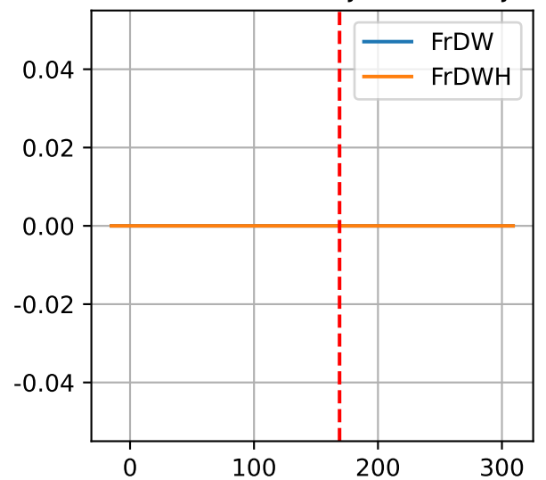
P1: ['FrDW', 'FrDWH', 'adjFrDW', 'adjFrDWH']
