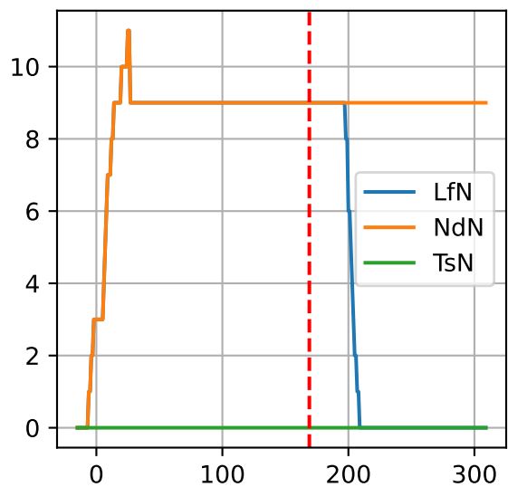
P1: ['LfN', 'NdN', 'TsN']
