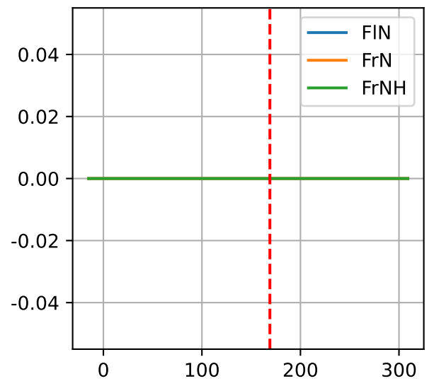
P1: ['FIN', 'FrN', 'FrNH']
