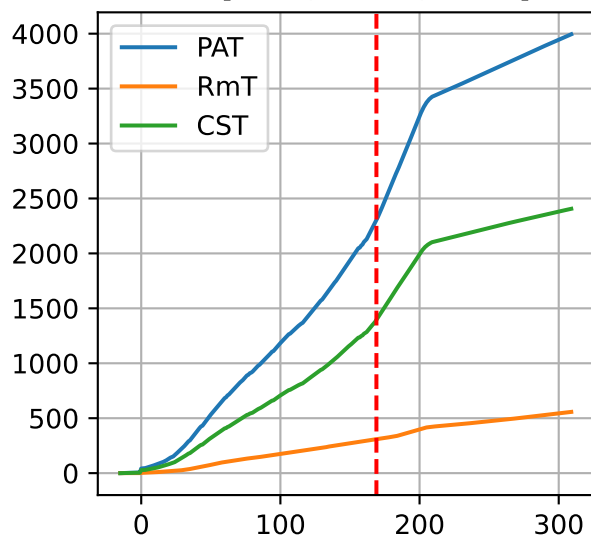
P1: ['PAT', 'RmT', 'CST']
