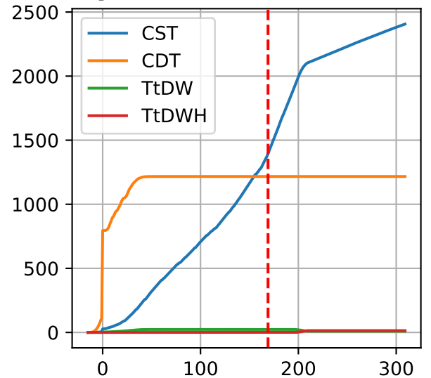
P1: ['CST', 'CDT', 'TtDW', 'TtDWH']
