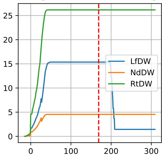
P1: ['LfDW', 'NdDW', 'RtDW']
