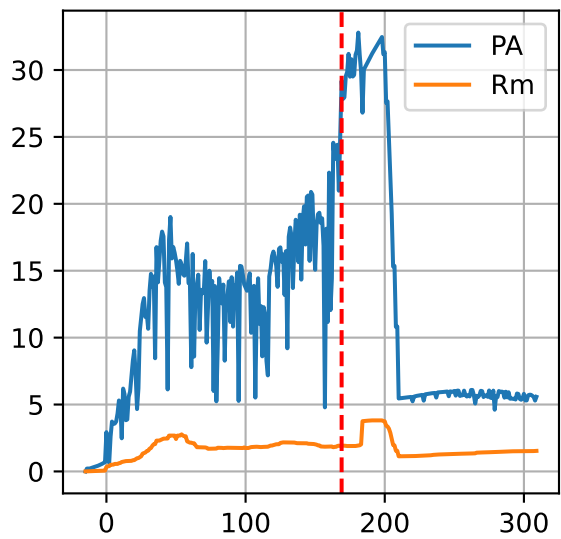
P1: ['PA', 'Rm']
