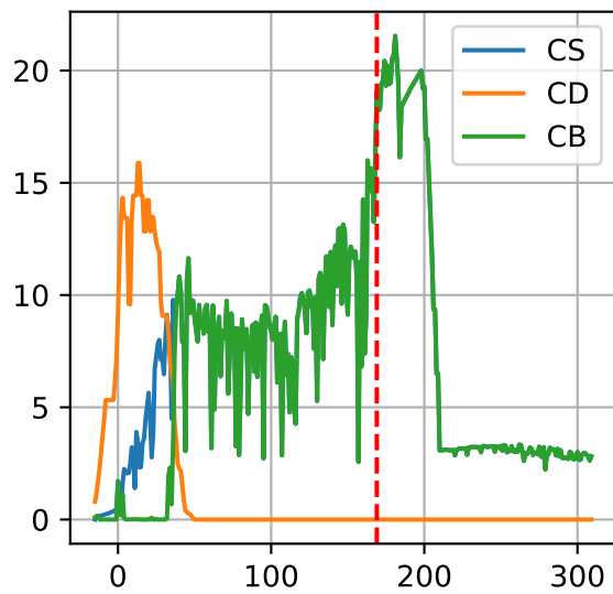
P1: ['CS', 'CD', 'CB']
