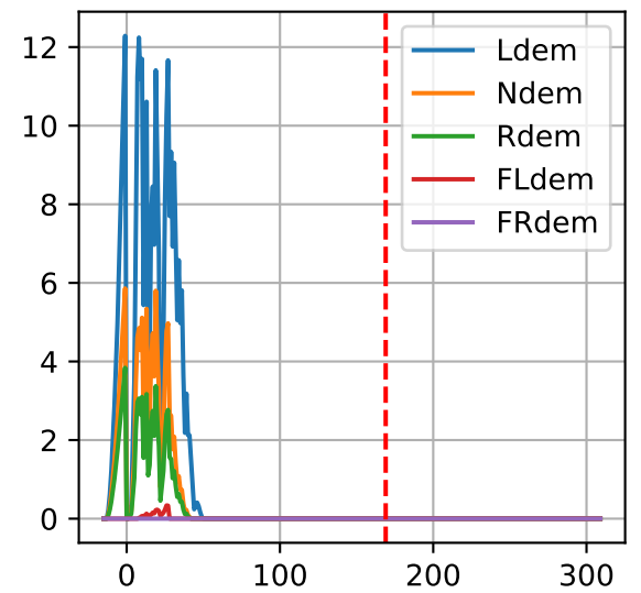
P1: ['Ldem', 'Ndem', 'Rdem', 'FLdem', 'FRdem']
