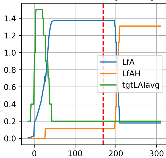
P1: ['LfA', 'LfAH', 'tgtLAlavg']
