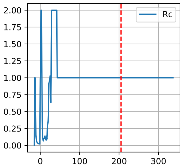
P2-2: ['Rc']
