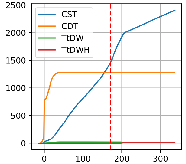
P2-3: ['CST', 'CDT', 'TtDW', 'TtDWH']
