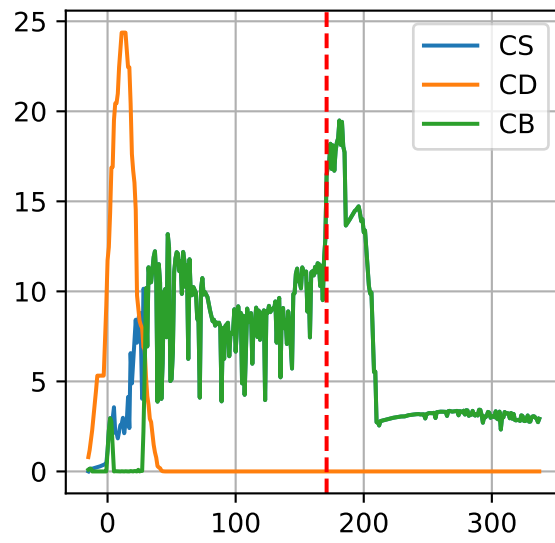
P2-3: ['CS', 'CD', 'CB']
