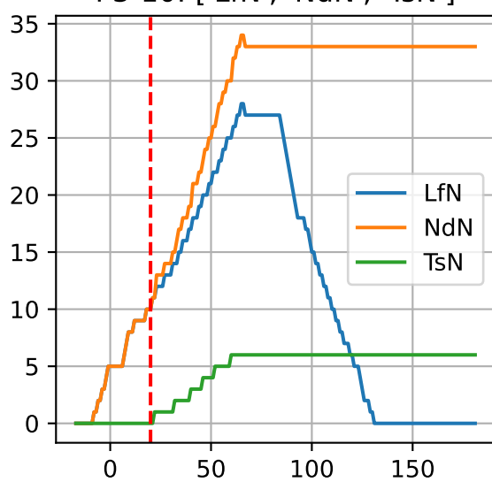
P3-10: ['LfN', 'NdN', 'TsN']
