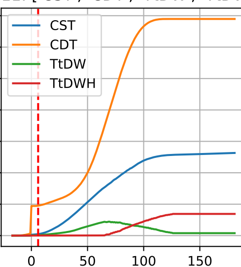
P3-11: ['CST', 'CDT', 'TtDW', 'TtDWH']
