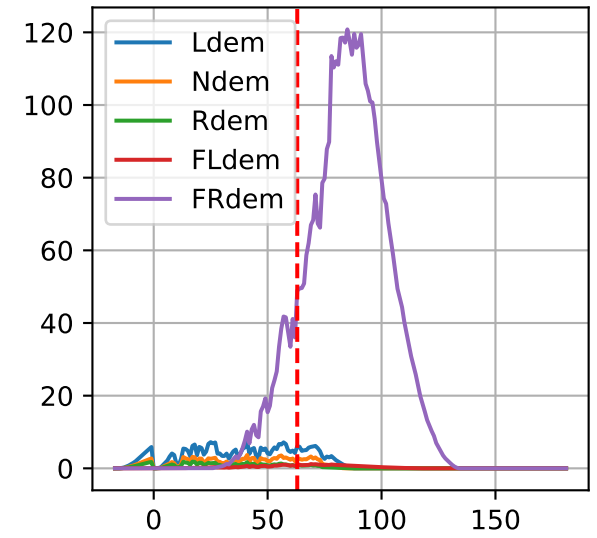
P3-11: ['Ldem', 'Ndem', 'Rdem', 'FLdem', 'FRdem']
