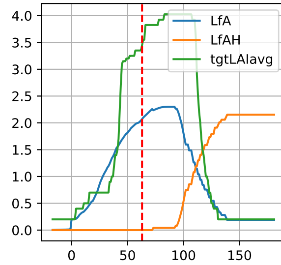
P3-11: ['LfA', 'LfAH', 'tgtLAlavg']
