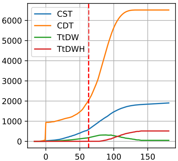
P3-11: ['CST', 'CDT', 'TtDW', 'TtDWH']
