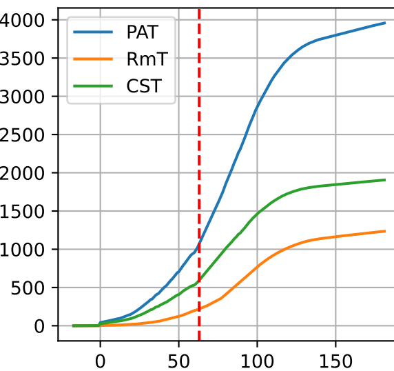
P3-11: ['PAT', 'RmT', 'CST']
