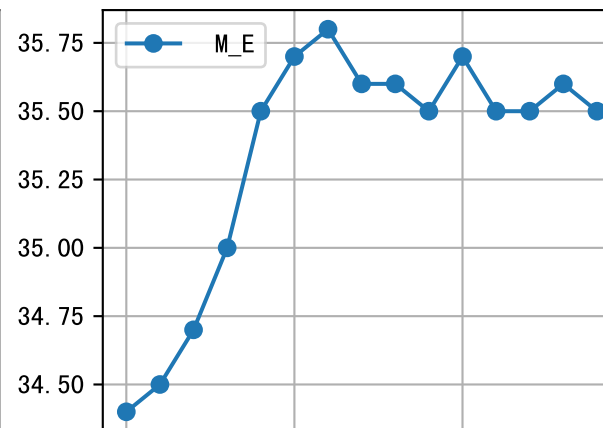
m=485, FV0=0
