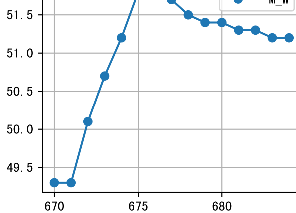
m=670, FV0=0
