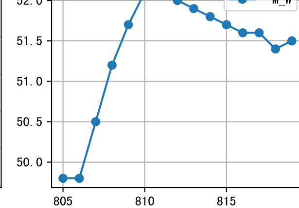
m=805, FV0=0
