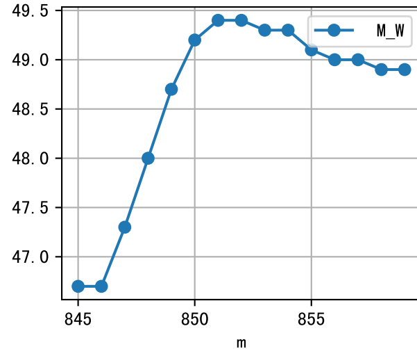
m=845, FV0=0
