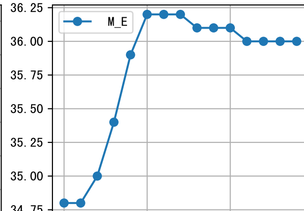
m=585, FV0=0
