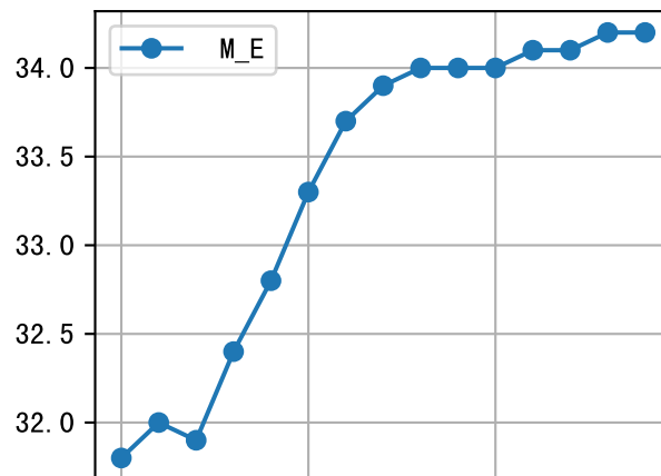
m=435, FV0=0
