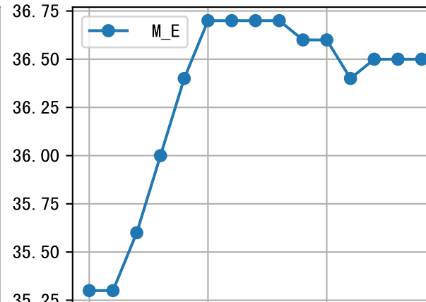
m=805, FV0=0
