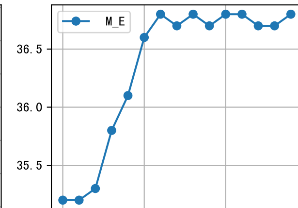
m=885, FV0=0
