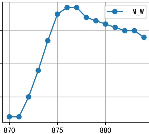
m=990, FV0=0
