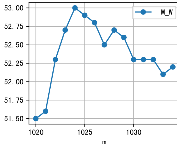
m=1020, FV0=0
