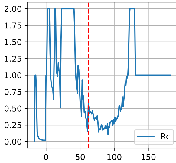
P3-14: ['Rc']
