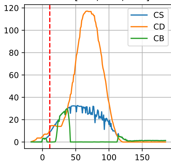
P3-1: ['CS', 'CD', 'CB']
