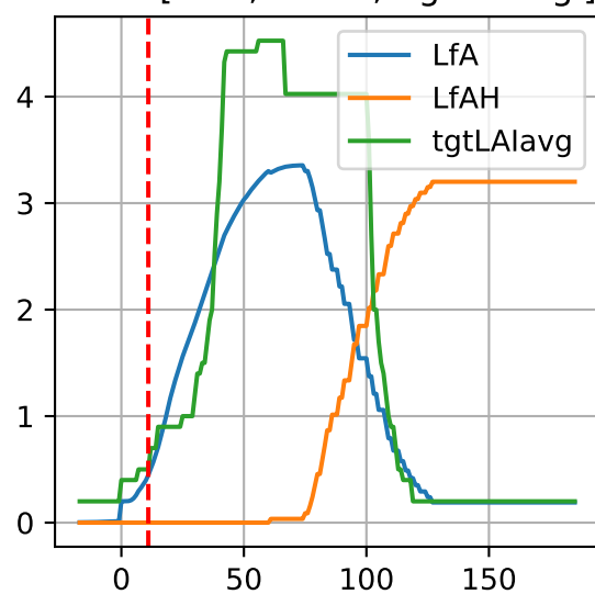
P3-1: ['LfA', 'LfAH', 'tgtLAlavg']
