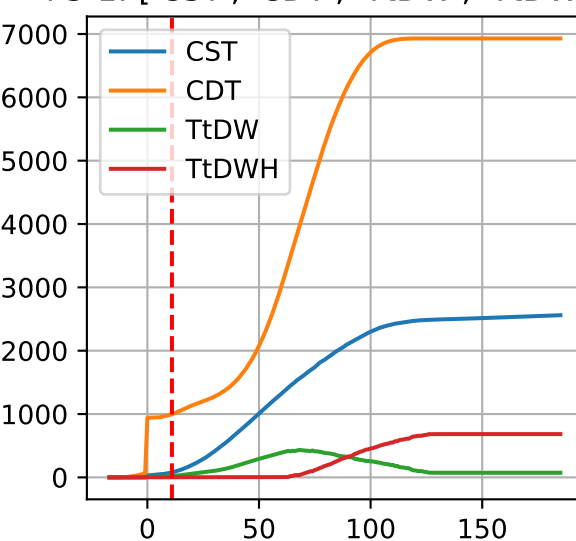
P3-1: ['CST', 'CDT', 'TtDW', 'TtDWH']
