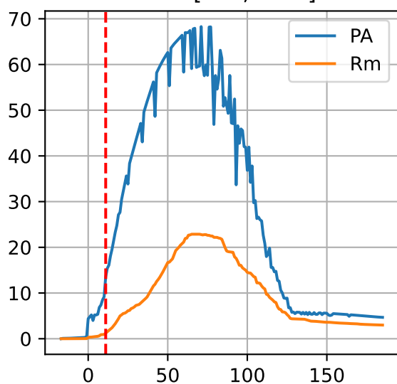
P3-1: ['PA', 'Rm']
