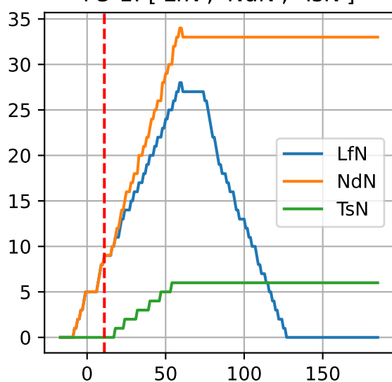
P3-1: ['LfN', 'NdN', 'TsN']
