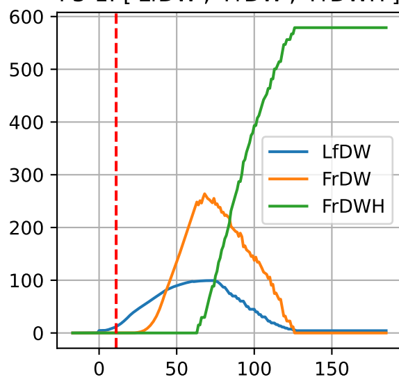
P3-1: ['LfDW', 'FrDW', 'FrDWH']
