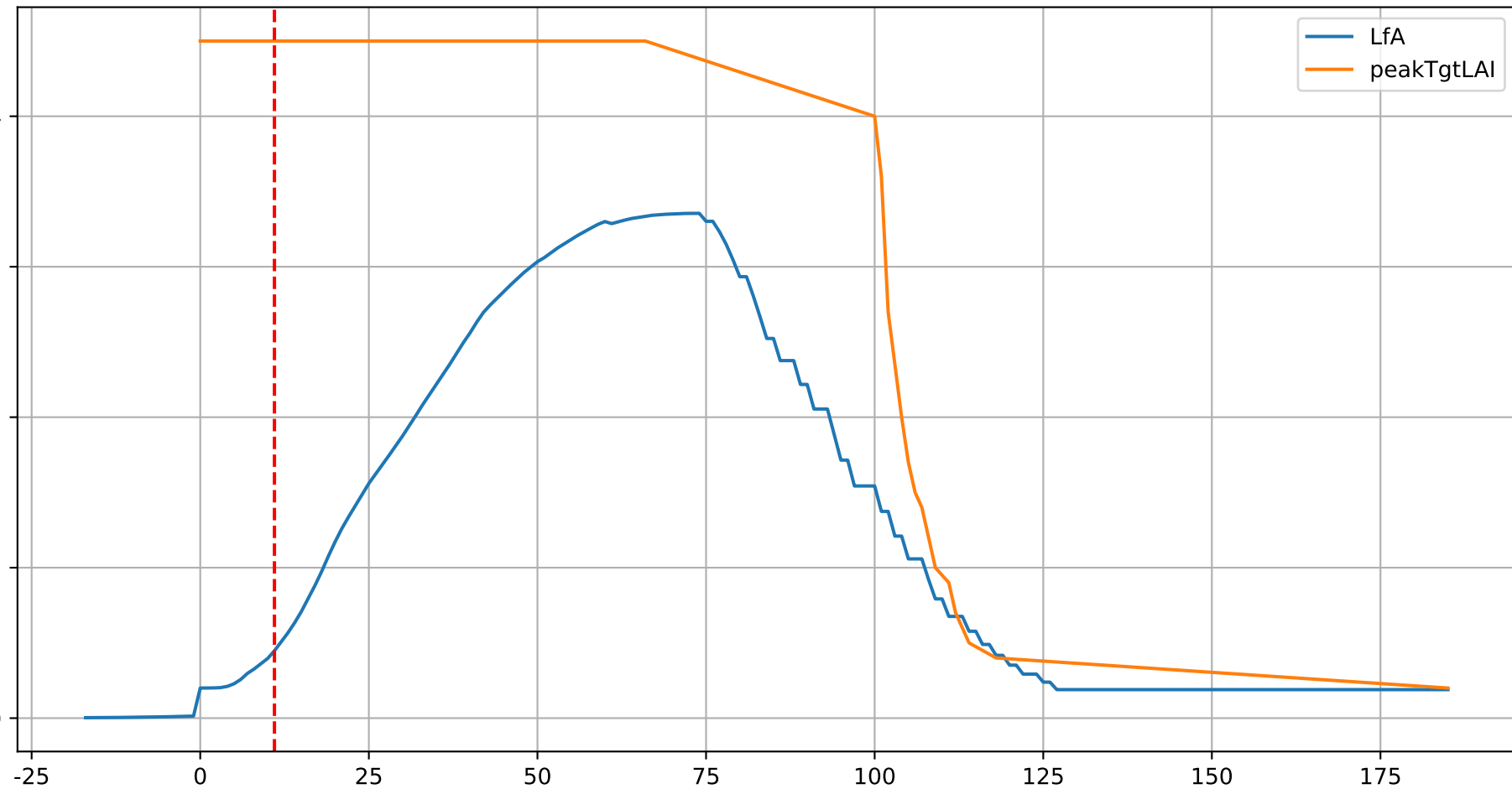
P3-1: ['LfA', 'peakTgtLAI']
