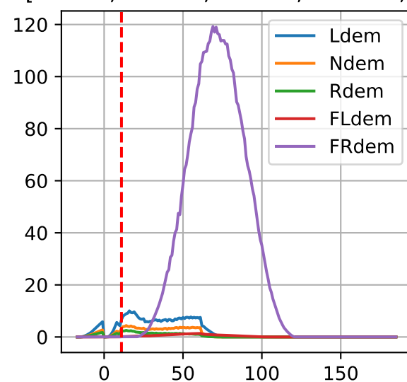
P3-1: ['Ldem', 'Ndem', 'Rdem', 'FLdem', 'FRdem']
