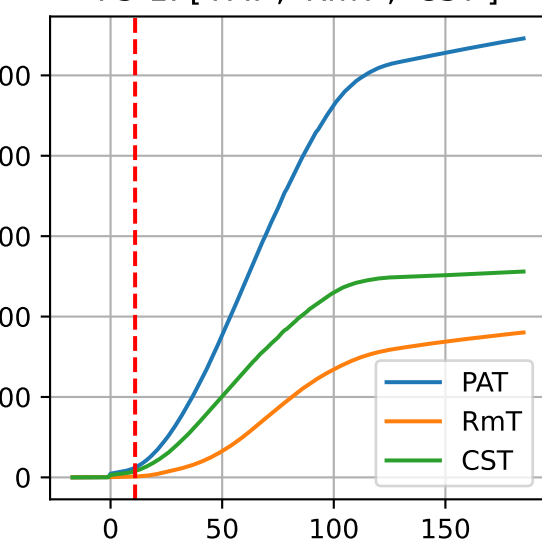
P3-1: ['PAT', 'RmT', 'CST']
