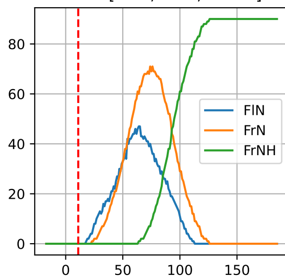
P3-1: ['FIN', 'FrN', 'FrNH']
