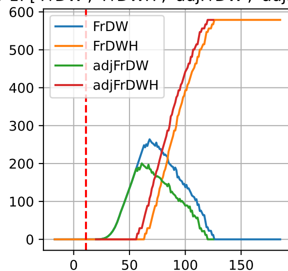
P3-1: ['FrDW', 'FrDWH', 'adjFrDW', 'adjFrDWH']
