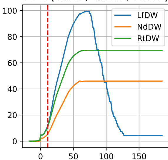
P3-1: ['LfDW', 'NdDW', 'RtDW']
