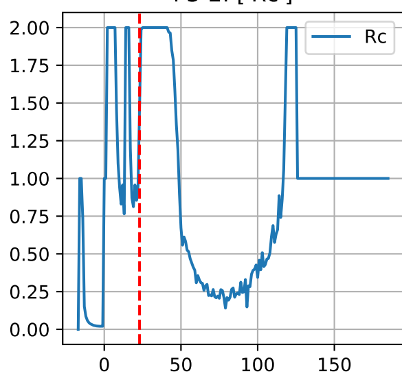
P3-2: ['Rc']
