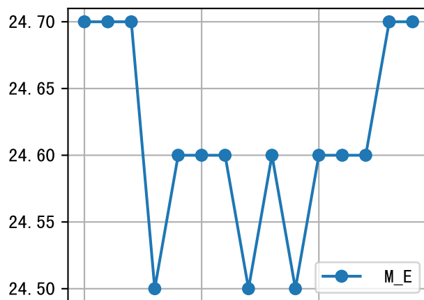
m=800, FV0=0
