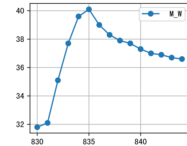
m=800,m FV0=0
