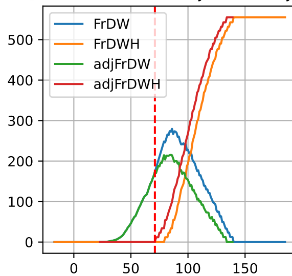
P3-4: ['FrDW', 'FrDWH', 'adjFrDW', 'adjFrDWH']
