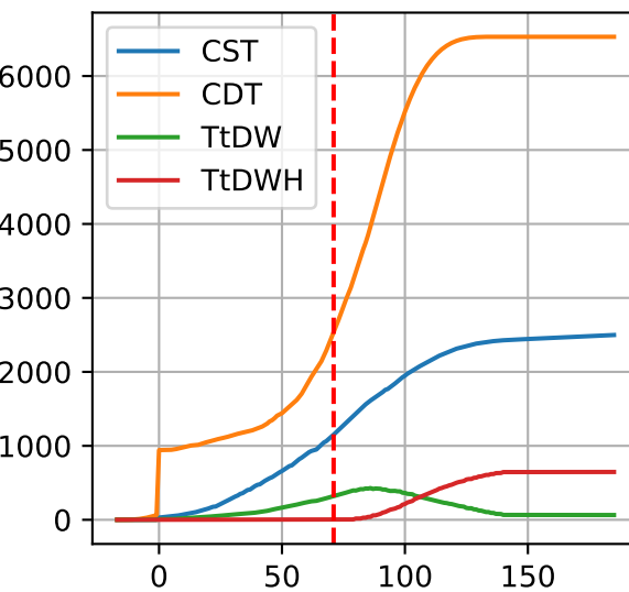
P3-4: ['CST', 'CDT', 'TtDW', 'TtDWH']
