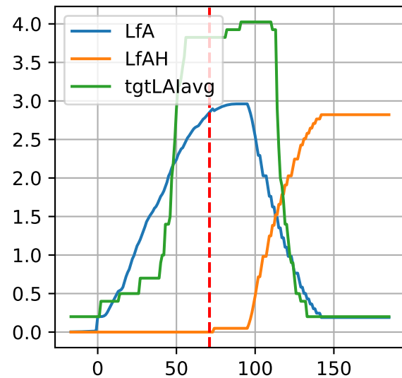
P3-4: ['LfA', 'LfAH', 'tgtLAlavg']
