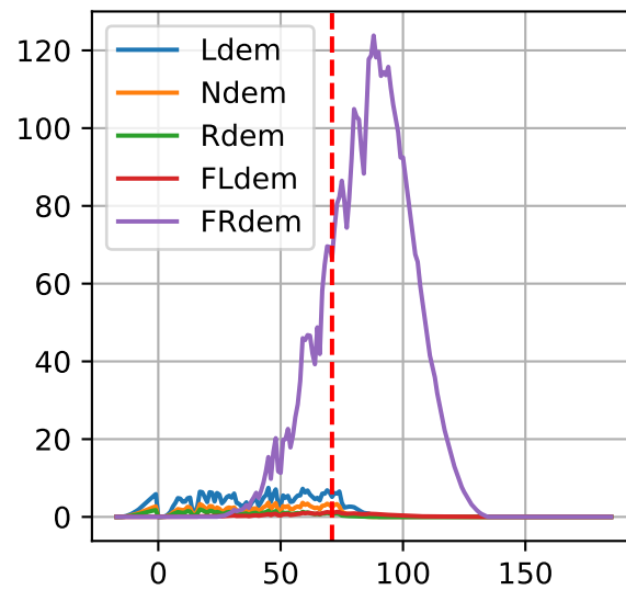
P3-4: ['Ldem', 'Ndem', 'Rdem', 'FLdem', 'FRdem']
