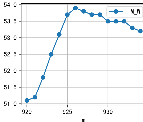
m=920, FV0=0
